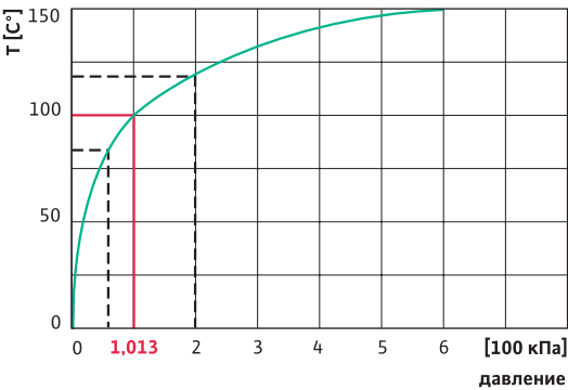
Температура кипения воды как функция давления
