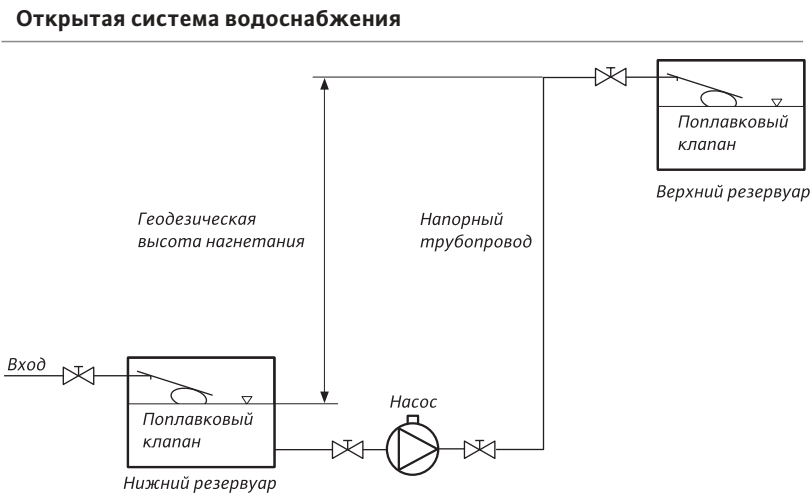
Насосная система для подачи воды на высоту
