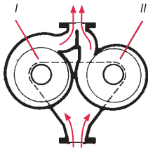
В работе оба насоса
