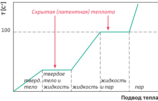
Изменение агрегатного состояния при повышении температуры
