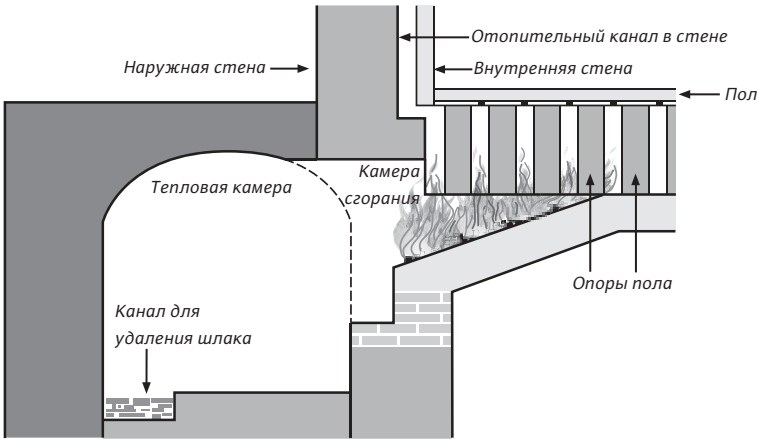
Система отопления "гипокауст" времен Римской Империи
