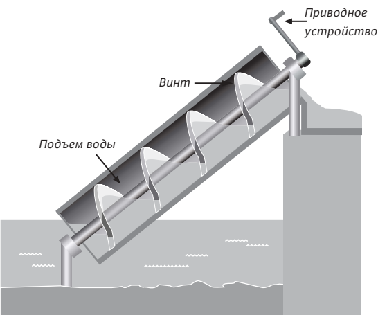
Архимедов винт
