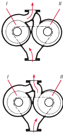
В работе насос I или насос II
