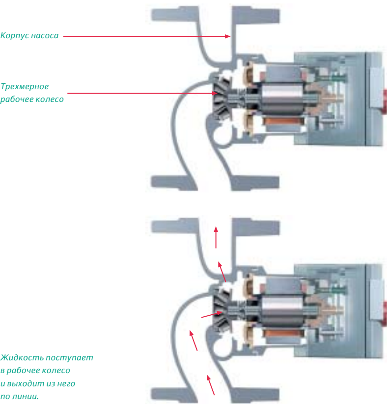
Разрез насоса с мокрым ротором
