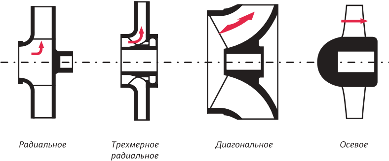
Типы рабочих колес
