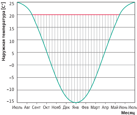
Температура наружного воздуха в зависимости от времени года
