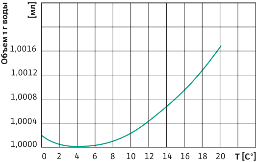
Изменение объема воды
