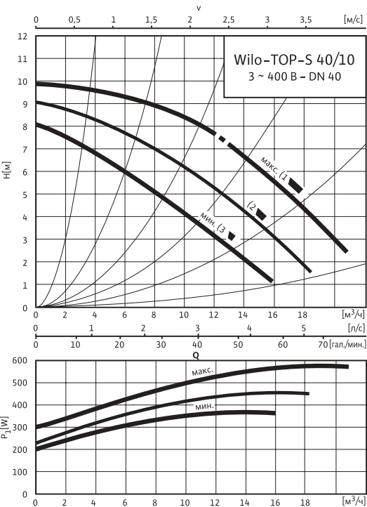
Характеристики Wilo-TOPI-S
